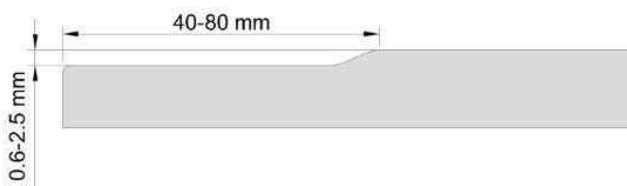
Muchie PRO – secțiune
